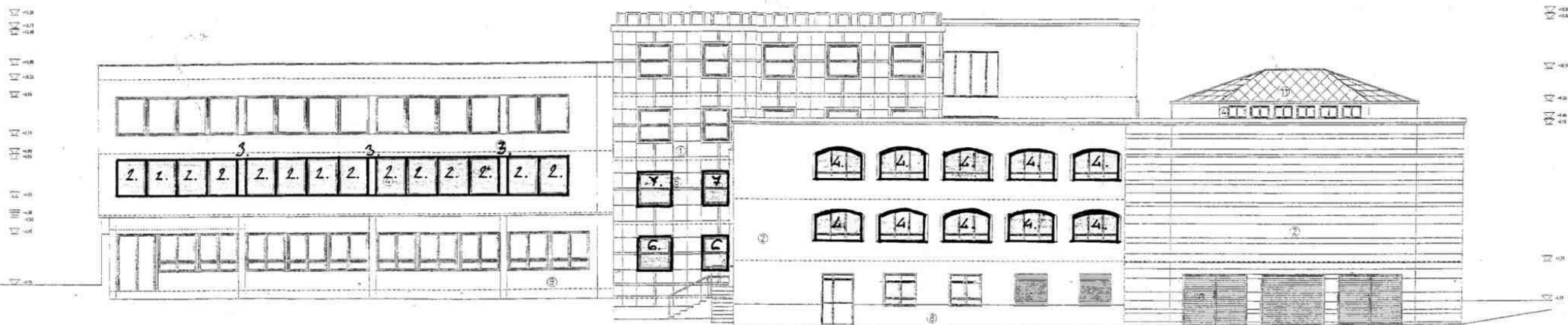
ÉSZAKI HOMLOKZAT
